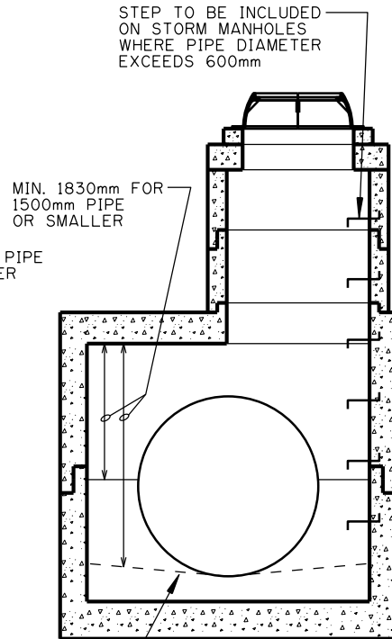
SECTION 'B-B'
