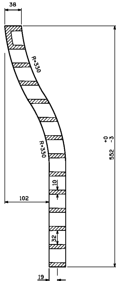
SECTION 'B-B'
