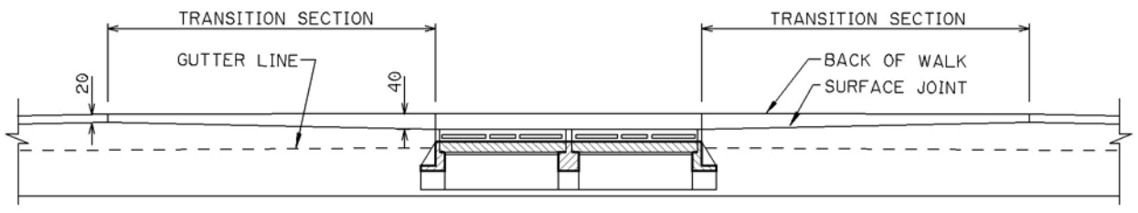
SECTION 'B-B'
