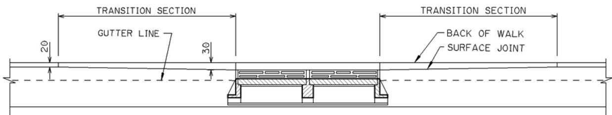
SECTION 'B-B'
